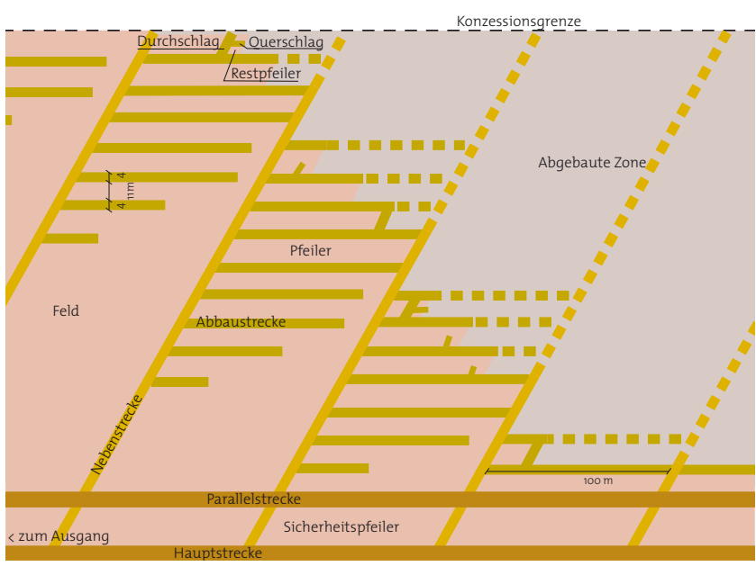
Draufsicht - Stollenbau
